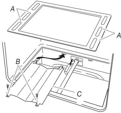
A. Bandeja del horno (levántela en el área mostrada para quitarla) B. Tornillos C. Partidor de llama
