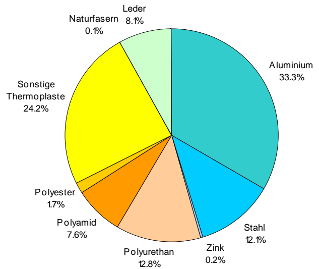
Skape Highback mit Fünfsternfuß (421 931 00) Bezugsstoffe werden je nach Material aufgetrennt in Kunststoffe oder Naturfasern.
