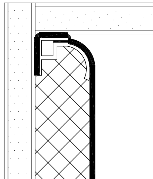
EDGE @ CEILING
