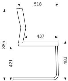
Freischwinger ohne Armlehne. Cantilever chair without armrests.
