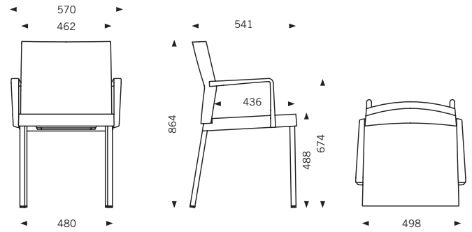
Vierfuß-Gestell mit Armlehne. / 4-legged frame with armrests.
