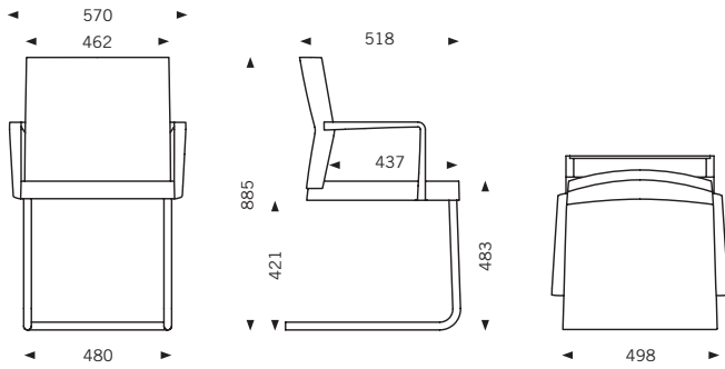
Freischwinger mit Armlehne. / Cantilever chair with armrests.
