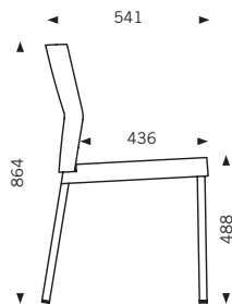
Vierfuß-Gestell ohne Armlehne. 4-legged frame without armrests.
