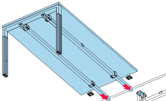
Variante C-/T-Fuss, Vollwange
