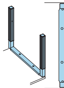
Montage von „4-Fuss mit Quadratrohr“ (T9).
