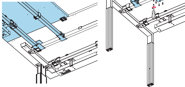
Variante C-/T-Fuss, Vollwange
