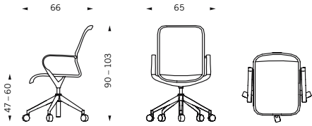
Filo. Fünfstern-Drehkreuz auf Rollen. Filo. Five-star base on castors.
