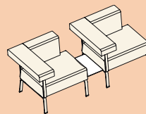
Verbindungsplatte. Connecting Panel. rechteckig / rectangular: B/W: 45, H: 30 cm dreieckig / triangular: B/W: 79, H: 43 cm
