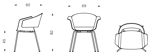
Rondo. Vierfuß-Gestell. Rondo. Four-leg frame.
