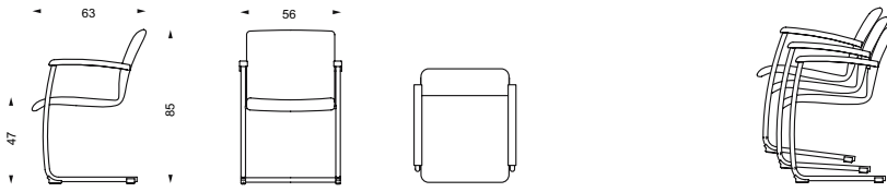
Bug. Freischwinger Bug. Cantilever Chair.
