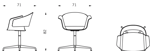
Rondo. Vierstern-Drehkreuz auf Gleitern. Rondo. Four-star base on glides.
