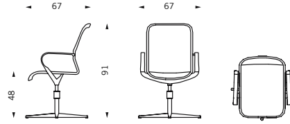
Filo. Vierstern-Drehkreuz auf Gleitern. Filo. Four-star base on glides.
