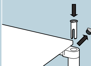
Einfache Montage einer Tischleuchte. Simple attachment of a table lamp.
