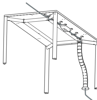
Kabelklammer einhängbar Suspended cable clamp
