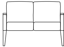
2800-20, Two Seat W=45", D=26½", H=32½", SH=18¾", AH=25"
