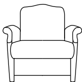
733-10, Chair W=30½", D=28¾", H=33" SH=18", AH=24"
