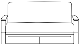
786□-37, Sofa W=86½", D=30", H=35" SH=18½", AH=25"
