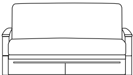
787-37, Sofa W=86½", D=30", H=35" SH=18½", AH=23½"
