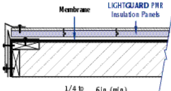
Detail Fig. 10A
