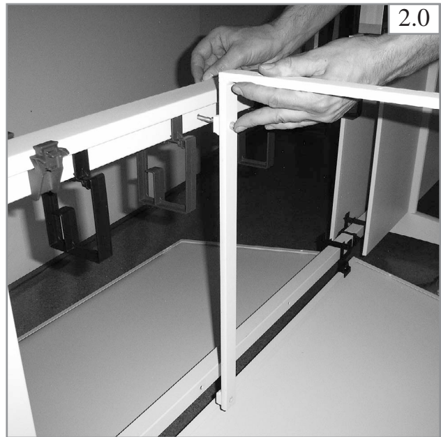
Boardträger an vorgegebener Position anschrauben. Screw board brackets into required position. Monter les supports à l'endroit prévu sur la structure.
