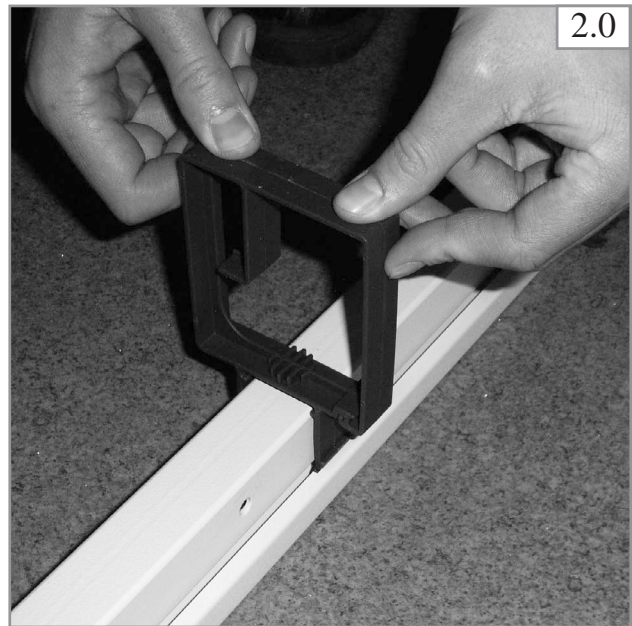
Kabelträger einklipsen. Attach cable brackets. Fixer les supports de câbles.
