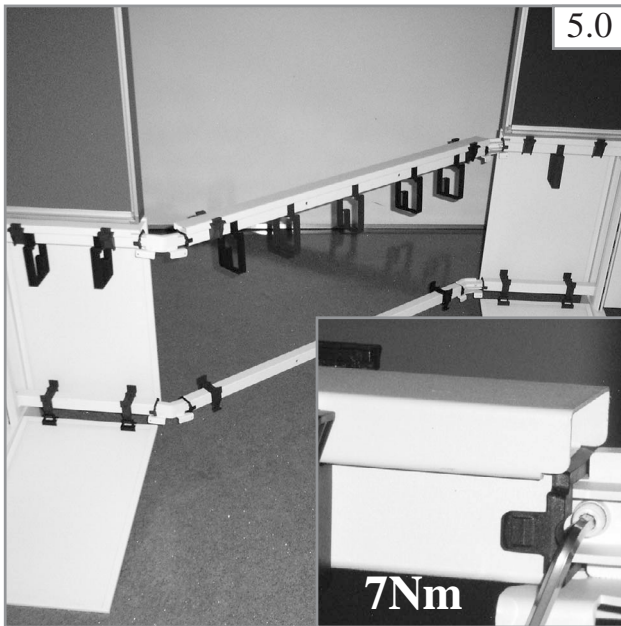
Verkettungsprofile in Verbinder stecken und festschrauben Insert junction profile into connectors and screw tight. Monter les profilés de liaison sur les connecteurs et visser.
