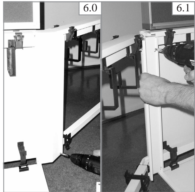
Blenden einhängen und verschrauben aussen/innen. Suspend covers and tighten outside/inside. Monter et visser les caches à l'intérieur et l'extérieur
