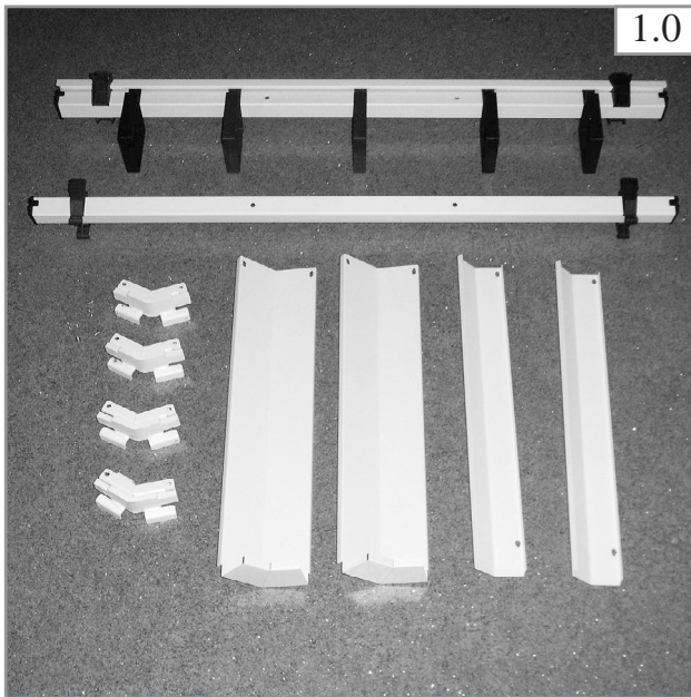
Verpackungsinhalt Verkettung 45°. 45° junction packaging contents Contenu de l'emballage Liaison 45°
