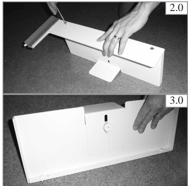
Befestigungsarm und Klemmwinkel an Bodenplatte schrauben. Screw fixing arm and clamp elements on to base shelf.
