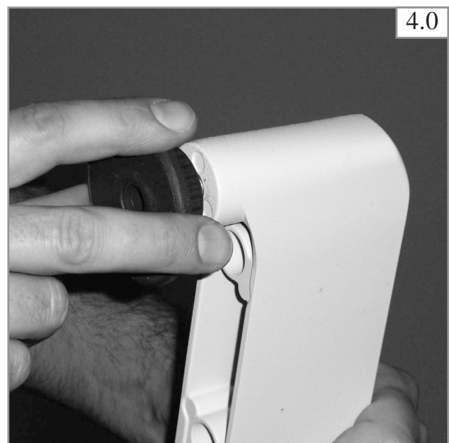
Stellschrauben in Ausleger schrauben Screw adjustable screws into extension Visser les vérins de réglage dans le pied.
