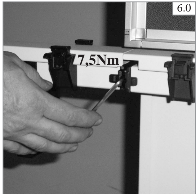
Verkettungsprofile festschrauben. Screw junction profile tight. Visser les profilés de liaison.
