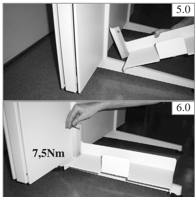
CPU-Halter einhängen und Alu-Klemmleiste festziehen. Suspend CPU holder and secure aluminium terminal block by pulling it tight. Accrocher le support UC au montant de la structure et serrer la plaque en alu.
