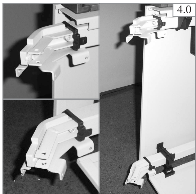
Verbinder in Profile einstecken. Insert connectors into profile. Introduire les connecteurs de liaison dans les profilés.
