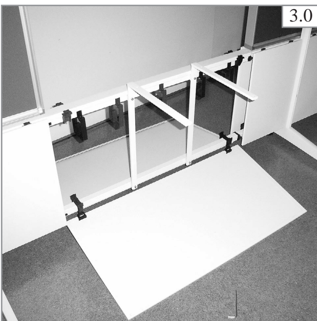
Fertig montierte Boardträger. Board brackets assembled. Vue des supports montés
