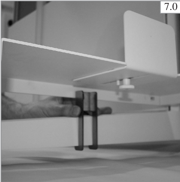
Haltehook einhängen. Suspend fixation. Accrocher fixation.
