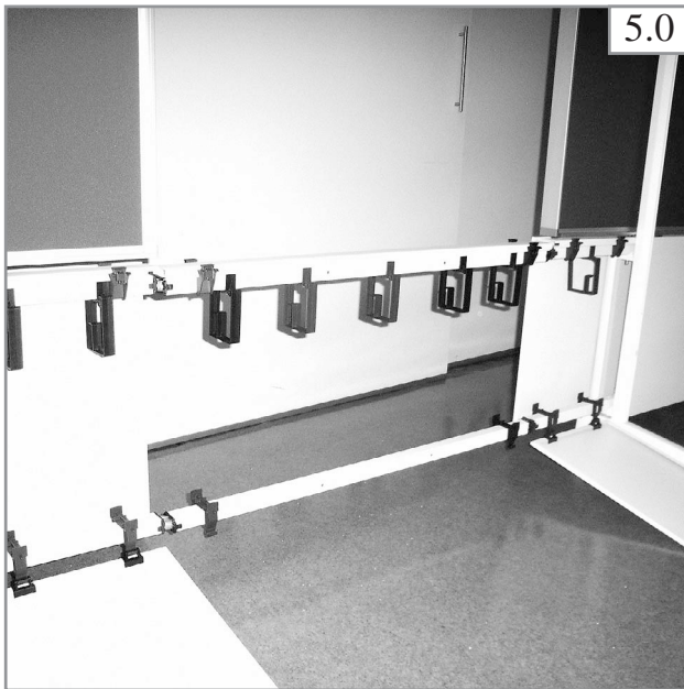
Verkettungsprofile in die Verbinder stecken. Insert junction profile into connectors. Monter les profilés de liaison sur les connecteurs.
