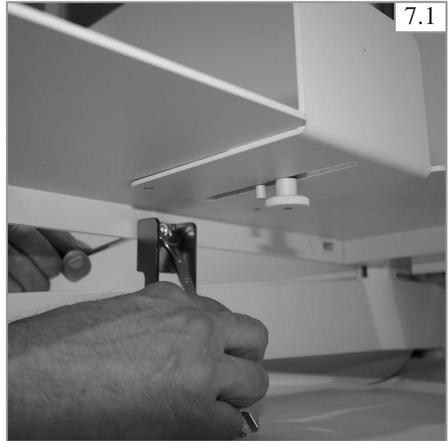
Haltehook festschrauben Fasten fixation Visser fixation
