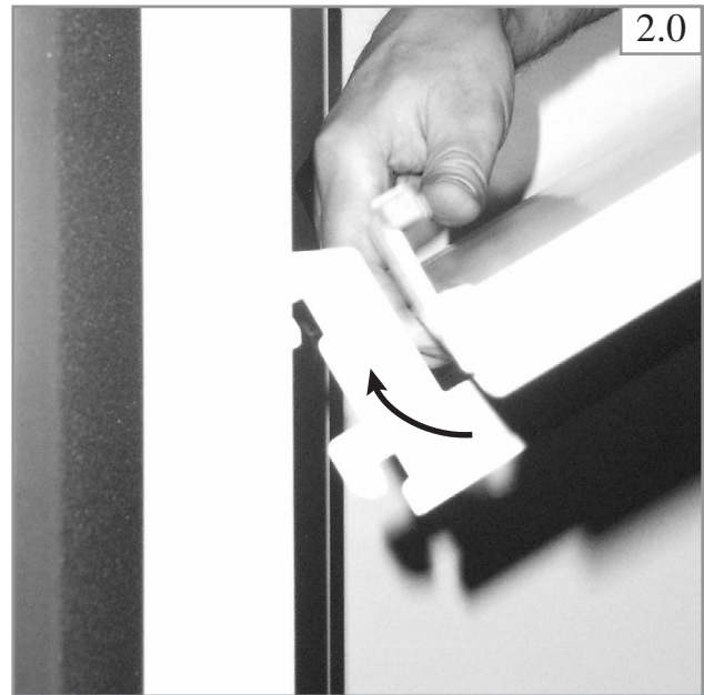
Board nach oben einhängen. Suspend board upwards. Introduire les crochets du support dans les montants
