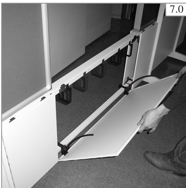
Kabelblenden einklipsen. Attach cable covers. Clipser les cache-câbles sur les profilés.
