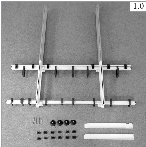
Verpackungsinhalt Gerüst (hier Typ 2+3) Frame packaging contents (type 2 + 3 shown here) Contenu de l'emballage Structure (ici type 2 + 3)
