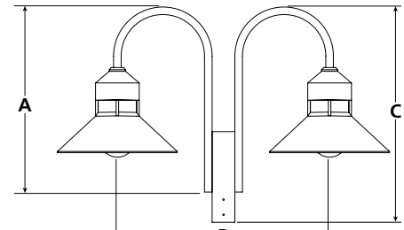
AA-30-AM2180/AA-31-AM2180
