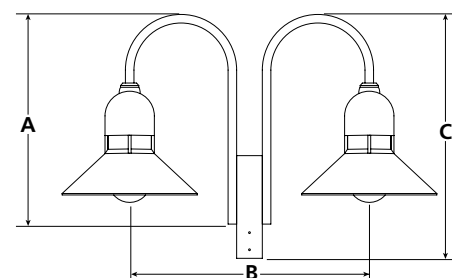
AA-130-AM2180/AA-131-AM2180
