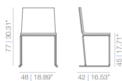
SLED BASE
