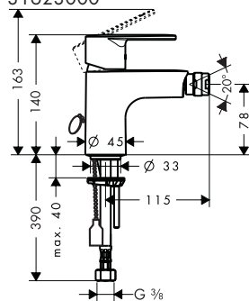
Talis E 2 31623000
