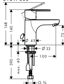
Talis E 2 31617000
