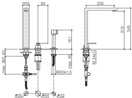
32 800 680 + 27 714 970 Two-hole mixer with individual flanges and handspray set, 9 1/4" spout projection Miscelatore monocomando a due fori con rosette separate e con gruppo doccetta lavello, sporgenza 9 1/4" Grifo mezclador con dos orificios con rosetas separadas y juego de grifo para cocina, saliente 9 1/4"
