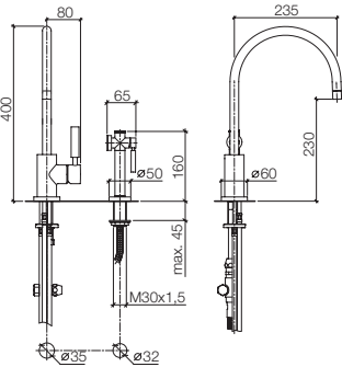
33 826 888 + 27 718 970 Single-lever mixer with handspray set, 9 1/4" spout projection Miscelatore monocomando con gruppo doccetta lavello, sporgenza 9 1/4" Mezclador monomando con juego de grifo para cocina, saliente 9 1/4"
