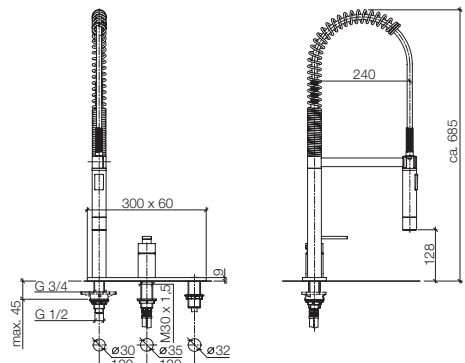
37 859 680 PREP SET Profi two-hole mixer, 9 1/2" spout projection, with Air Switch (operating button) Miscelatore monocomando a due fori professionale, sporgenza 9 1/2", con Air Switch Grifo mezclador profesional con dos orificios, saliente 9 1/2", con Air Switch
