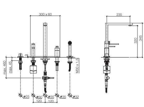
37 847 680 + 10 711 970 UNI SET Two-hole mixer with handspray set, 9 1/4" spout projection + strainer remote control Miscelatore monocomando a due fori con gruppo doccetta lavello, sporgenza 9 1/4" + Comando piletta ad eccentrico Grifo mezclador con dos orificios con juego de grifo para cocina, saliente 9 1/4" + Accionamiento excéntrico
