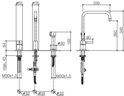
32 815 625 + 27 719 970 Two-hole mixer with handspray set, 9 1/4" spout projection Miscelatore monocomando a due fori con gruppo doccetta lavello, sporgenza 9 1/4" Grifo mezclador con dos orificios con juego de grifo para cocina, saliente 9 1/4"
