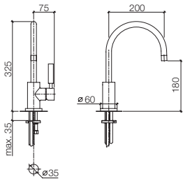
33 800 888 Single-lever mixer, 7 7/8" spout projection Miscelatore monocomando, sporgenza 7 7/8" Mezclador monomando, saliente 7 7/8"
