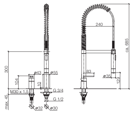
32 835 680 Profi two-hole mixer, 9 1/2" spout projection Miscelatore monocomando a due fori professionale, sporgenza 9 1/2" Grifo mezclador profesional con dos orificios, saliente 9 1/2"
