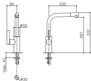
33 800 791 Single-lever mixer with lever on left, 9 1/4" spout projection Miscelatore monocomando con leva a sinistra, sporgenza 9 1/4" Mezclador monomando con palanca a la izquierda, saliente 9 1/4"
