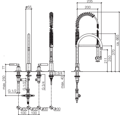
20 815 882 + 27 780 970 Three-hole mixer with Profi spray set, 9 1/4" spout projection Batteria tre fori con batteria doccetta professionale, sporgenza 9 1/4" Grifo mezclador con tres orificios con juego de grifo profesional tipo ducha, saliente 9 1/4"
