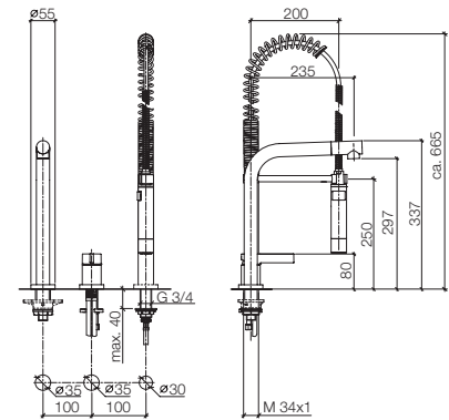
32 800 790 + 27 789 970 Two-hole mixer with individual flanges and Profi spray set, 9 1/4" spout projection Miscelatore monocomando a due fori con rosette separate e batteria doccetta professionale, sporgenza 9 1/4" Grifo mezclador con dos orificios con rosetas separadas y juego de grifo profesional tipo ducha, saliente 9 1/4"
