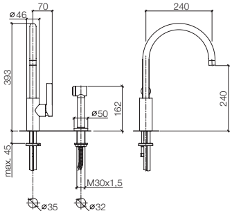
33 826 875 / 33 826 876 + 27 719 970 Single-lever mixer with handspray set, 9 1/2" spout projection Miscelatore monocomando con gruppo doccetta lavello, sporgenza 9 1/2" Mezclador monomando con juego de grifo para cocina, saliente 9 1/2"
