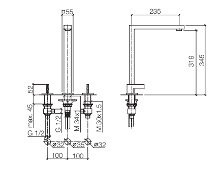
20 810 680 Three-hole mixer with individual flanges, 9 1/4" spout projection Batteria tre fori con rosette separate, sporgenza 9 1/4" Grifo mezclador con tres orificios con rosetas separadas, saliente 9 1/4"
