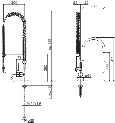
33 880 889 Profi single-lever mixer with lever on left, 9 1/4" spout projection Miscelatore monocomando professionale con leva a sinistra, sporgenza 9 1/4" Mezclador monomando profesional con palanca a la izquierda, saliente 9 1/4"
