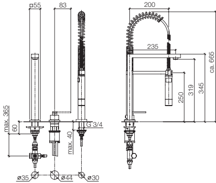
32 800 680 + 27 784 970 Two-hole mixer with individual flanges and Profi spray set, 9 1/4" spout projection Miscelatore monocomando a due fori con rosette separate e batteria doccetta professionale, sporgenza 9 1/4" Grifo mezclador con dos orificios con rosetas separadas y juego de grifo profesional tipo ducha, saliente 9 1/4"
