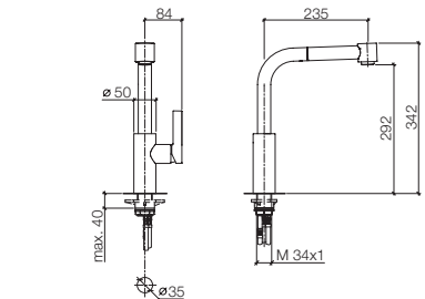
33 870 790 Single-lever mixer with pull-out spray set, 9 1/4" spout projection Miscelatore monocomando con doccetta estraibile, sporgenza 9 1/4" Mezclador monomando con ducha extraíble, saliente 9 1/4"
