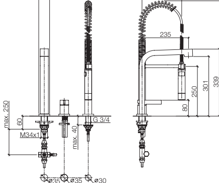
32 800 795 + 27 784 970 Two-hole mixer with individual flanges and Profi spray set, 9 1/4" spout projection Miscelatore monocomando a due fori con rosette separate e batteria doccetta professionale, sporgenza 9 1/4" Grifo mezclador con dos orificios con rosetas separadas y juego de grifo profesional tipo ducha, saliente 9 1/4"
