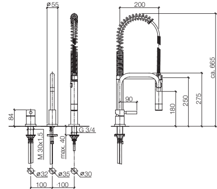
32 800 625 + 27 789 970 Two-hole mixer with Profi spray set, 7 7/8" spout projection Miscelatore monocomando a due fori con batteria doccetta professionale, sporgenza 7 7/8" Grifo mezclador con dos orificios con juego de grifo profesional tipo ducha, saliente 7 7/8"
