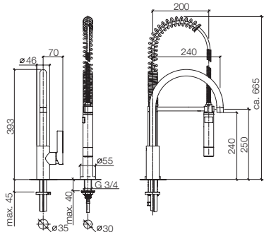
33 826 875 / 33 826 876 + 27 789 970 Single-lever mixer with Profi spray set, 9 1/2" spout projection Miscelatore monocomando con batteria doccetta professionale, sporgenza 9 1/2" Mezclador monomando con juego de grifo profesional tipo ducha, saliente 9 1/2"
