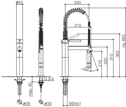
33 826 625 + 27 789 970 Single-lever mixer with Profi spray set, 8 1/2" spout projection Miscelatore monocomando con batteria doccetta professionale, sporgenza 8 1/2" Mezclador monomando con juego de grifo profesional tipo ducha, saliente 8 1/2"
