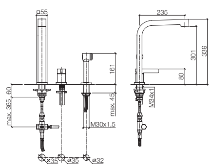
32 800 795 + 27 714 970 Two-hole mixer with individual flanges and handspray set, 9 1/4" spout projection Miscelatore monocomando a due fori con rosette separate e con gruppo doccetta lavello, sporgenza 9 1/4" Grifo mezclador con dos orificios con rosetas separadas y juego de grifo para cocina, saliente 9 1/4"
