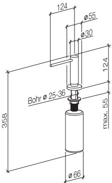
82 436 970 Deck-mounted liquid soap dispenser with flange Dispenser per detersivo liquido da incasso con rosetta Dosificador de lavavajillas encastrable con roseta
