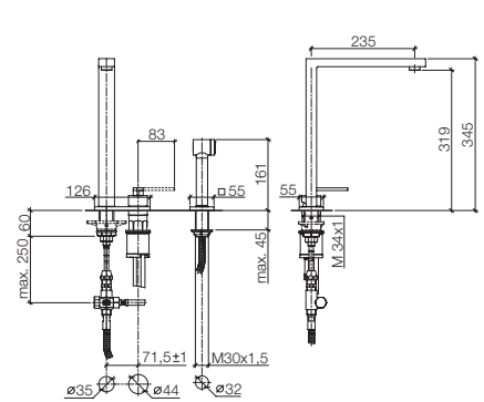
32 843 680 + 27 714 970 Two-hole mixer with cover plate and handspray set, 9 1/4" spout projection Miscelatore monocomando a due fori con piastra di copertura e con gruppo doccetta lavello, sporgenza 9 1/4" Grifo mezclador con dos orificios con cubierta y juego de grifo para cocina, saliente 9 1/4"
