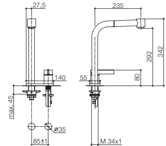
32 800 790 Two-hole mixer with individual flanges, 9 1/4" spout projection Miscelatore monocomando a due fori con rosette separate, sporgenza 9 1/4" Grifo mezclador con dos orificios con rosetas separadas, saliente 9 1/4"
