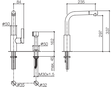
33 826 790 + 27 719 970 Single-lever mixer with handspray set, 9 1/4" spout projection Miscelatore monocomando con gruppo doccetta lavello, sporgenza 9 1/4" Mezclador monomando con juego de grifo para cocina, saliente 9 1/4"
