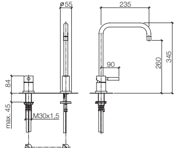
32 815 625 Two-hole mixer, 9 1/4" spout projection Miscelatore monocomando a due fori, sporgenza 9 1/4" Grifo mezclador con dos orificios, saliente 9 1/4"
