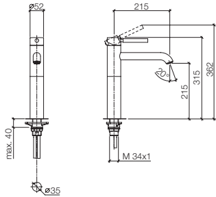
33 800 625 Single-lever mixer, 8 1/2" spout projection Miscelatore monocomando, sporgenza 8 1/2" Mezclador monomando, saliente 8 1/2"
