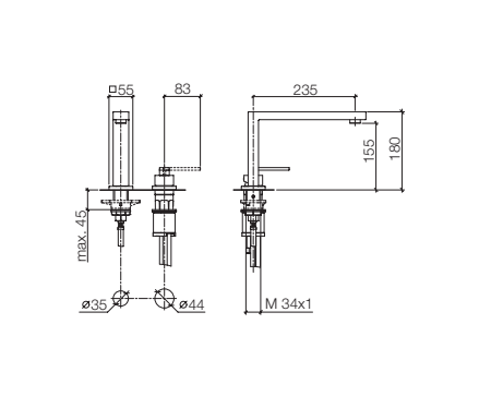
32 812 680 Two-hole mixer with individual flanges, 9 1/4" spout projection Miscelatore monocomando a due fori con rosette separate, sporgenza 9 1/4" Grifo mezclador con dos orificios con rosetas separadas, saliente 9 1/4"
