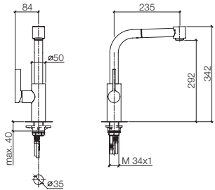
33 870 791 Single-lever mixer with pull-out spray set, lever on left, 9 1/4" spout projection Miscelatore monocomando con doccetta estraibile, leva a sinistra, sporgenza 9 1/4" Mezclador monomando con ducha extraíble, palanca a la izquierda, saliente 9 1/4"
