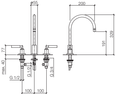
20 712 882 Three-hole mixer, 7 7/8" spout projection Batteria tre fori, sporgenza 7 7/8" Grifo mezclador con tres orificios, saliente 7 7/8"
