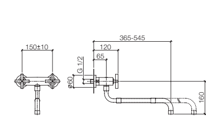
31 151 892 Wall-mounted bridge mixer with extendable spout, 14 3/8-21 1/2" spout projection Batteria arcata montaggio a muro con bocca estraibile, sporgenza 14 3/8-21 1/2" Grifo mezclador de puente montaje a pared con caño telescópico, saliente 14 3/8-21 1/2"
