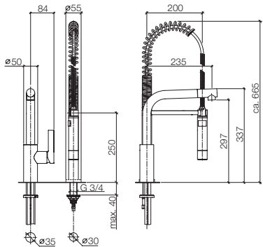
33 826 790 + 27 789 970 Single-lever mixer with Profi spray set, 9 1/4" spout projection Miscelatore monocomando con batteria doccetta professionale, sporgenza 9 1/4" Mezclador monomando con juego de grifo profesional tipo ducha, saliente 9 1/4"
