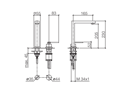
32 805 680 BAR TAP Two-hole mixer with individual flanges, 6 1/2" spout projection Miscelatore monocomando a due fori con rosette separate, sporgenza 6 1/2" Grifo mezclador con dos orificios con rosetas separadas, saliente 6 1/2"
