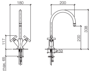
22 021 892 Single-hole mixer, 7 7/8" spout projection Batteria monoforo, sporgenza 7 7/8" Grifo mezclador con un orificio, saliente 7 7/8"
