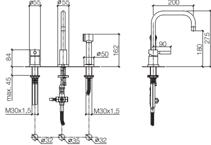
32 800 625 + 27 719 970 Two-hole mixer with handspray set, 7 7/8" spout projection Miscelatore monocomando a due fori con gruppo doccetta lavello, sporgenza 7 7/8" Grifo mezclador con dos orificios con juego de grifo para cocina, saliente 7 7/8"
