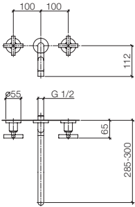
36 818 892 Wall-mounted mixer, 11 3/4" spout projection Batteria tre fori lavello incasso a muro, sporgenza 11 3/4" Bateria de pared para fregadero, saliente 11 3/4"
