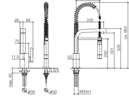
33 826 795 + 27 784 970 Single-lever mixer with Profi spray set, 9 1/4" spout projection Miscelatore monocomando con batteria doccetta professionale, sporgenza 9 1/4" Mezclador monomando con juego de grifo profesional tipo ducha, saliente 9 1/4"
