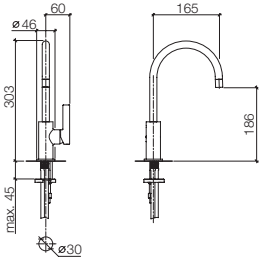
33 805 875 BAR TAP Single-lever mixer, 6 1/2" spout projection Miscelatore monocomando, sporgenza 6 1/2" Mezclador monomando, saliente 6 1/2"
