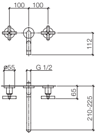
36 817 892 Wall-mounted mixer, 8 7/8" spout projection Batteria tre fori lavello incasso a muro, sporgenza 8 7/8" Bateria de pared para fregadero, saliente 8 7/8"
