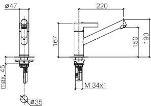
33 800 760 Single-lever mixer, 8 5/8" spout projection Miscelatore monocomando, sporgenza 8 5/8" Mezclador monomando, saliente 8 5/8"
