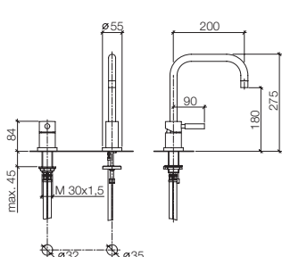
32 800 625 Two-hole mixer, 7 7/8" spout projection Miscelatore monocomando a due fori, sporgenza 7 7/8" Grifo mezclador con dos orificios, saliente 7 7/8"
