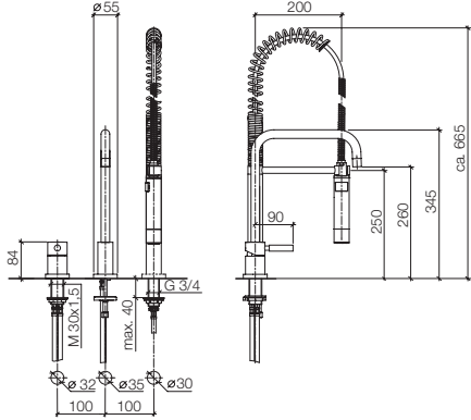
32 815 625 + 27 789 970 Two-hole mixer with Profi spray set, 9 1/4" spout projection Miscelatore monocomando a due fori con batteria doccetta professionale, sporgenza 9 1/4" Grifo mezclador con dos orificios con juego de grifo profesional tipo ducha, saliente 9 1/4"
