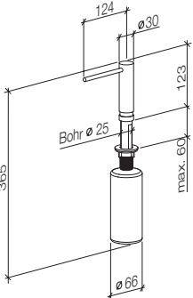
82 426 970 Deck-mounted liquid soap dispenser without flange Dispenser per detersivo liquido da incasso senza rosetta Dosificador de lavavajillas encastrable sin roseta
