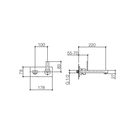
36 820 680 Wall-mounted single-lever mixer with cover plate, 8 5/8" spout projection Miscelatore a muro con piastra di copertura, sporgenza 8 5/8" Mezclador de pared con cubierta, saliente 8 5/8"
