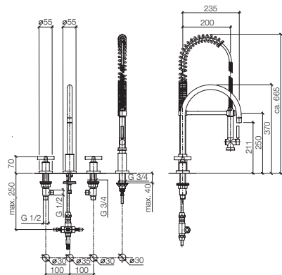
20 815 892 + 27 780 970 Three-hole mixer with Profi spray set, 9 1/4" spout projection Batteria tre fori con batteria doccetta professionale, sporgenza 9 1/4" Grifo mezclador con tres orificios con juego de grifo profesional tipo ducha, saliente 9 1/4"
