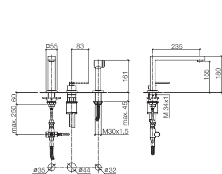
32 812 680 + 27 714 970 Two-hole mixer with individual flanges and handspray set, 9 1/4" spout projection Miscelatore monocomando a due fori con gruppo doccetta lavello, sporgenza 9 1/4" Grifo mezclador con dos orificios con juego de grifo para cocina, saliente 9 1/4"
