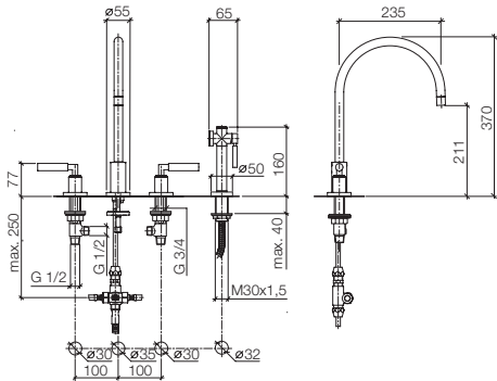
20 815 882 + 27 718 970 Three-hole mixer with handspray set, 9 1/4" spout projection Batteria tre fori con gruppo doccetta lavello, sporgenza 9 1/4" Grifo mezclador con tres orificios con juego de grifo para cocina, saliente 9 1/4"
