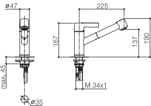
33 870 760 Single-lever mixer with pull-out spray set, 8 5/8" spout projection Miscelatore monocomando con doccetta estraibile, sporgenza 8 5/8" Mezclador monomando con ducha extraible, saliente 8 5/8"
