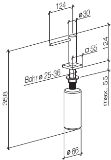
82 438 970 Deck-mounted liquid soap dispenser with flange Dispenser per detersivo liquido da incasso con rosetta Dosificador de lavavajillas encastrable con roseta
