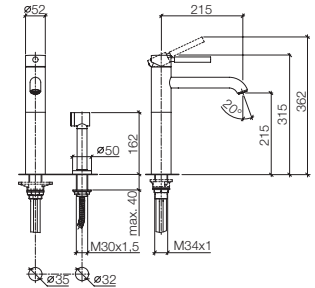
33 826 625 + 27 719 970 Single-lever mixer with handspray set, 8 1/2" spout projection Miscelatore monocomando con gruppo doccetta lavello, sporgenza 8 1/2" Mezclador monomando con juego de grifo para cocina, saliente 8 1/2"
