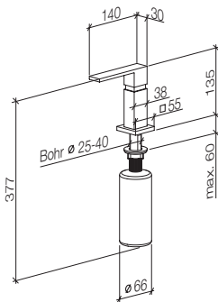
82 437 970 Deck-mounted liquid soap dispenser with flange Dispenser per detersivo liquido da incasso con rosetta Dosificador de lavavajillas encastrable con roseta
