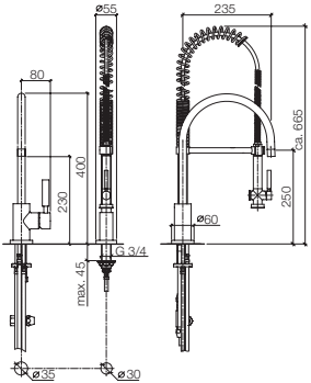
33 826 888 + 27 780 970 Single-lever mixer with Profi spray set, 9 1/4" spout projection Miscelatore monocomando con batteria doccetta professionale, sporgenza 9 1/4" Mezclador monomando con juego de grifo profesional tipo ducha, saliente 9 1/4"
