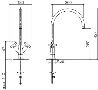
22 834 892 Single-hole mixer with extended shank, 10 1/4" spout projection Batteria monoforo con base rialzata, sporgenza 10 1/4" Grifo mezclador con un orificio con base elevada, saliente 10 1/4"
