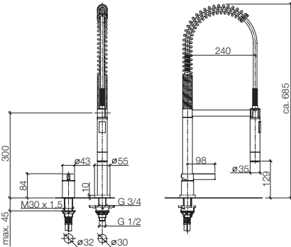
32 835 875 Profi two-hole mixer, 9 1/2" spout projection Miscelatore monocomando a due fori professionale, sporgenza 9 1/2" Grifo mezclador profesional con dos orificios, saliente 9 1/2"
