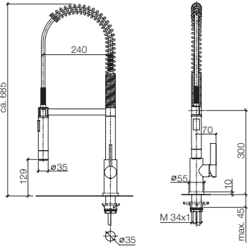
33 860 875 Profi single-lever mixer, 9 1/2" spout projection Miscelatore monocomando professionale, sporgenza 9 1/2" Mezclador monomando profesional, saliente 9 1/2"
