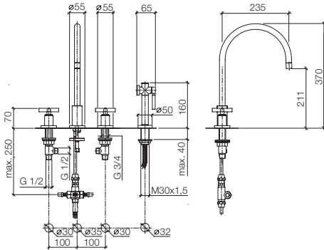
20 815 892 + 27 718 970 Three-hole mixer with handspray set, 9 1/4" spout projection Batteria tre fori con gruppo doccetta lavello, sporgenza 9 1/4" Grifo mezclador con tres orificios con juego de grifo para cocina, saliente 9 1/4"
