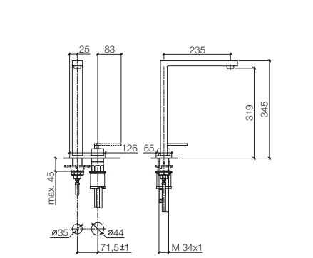
32 843 680 Two-hole mixer with cover plate, 9 1/4" spout projection Miscelatore monocomando a due fori con piastra di copertura, sporgenza 9 1/4" Grifo mezclador con dos orificios con cubierta, saliente 9 1/4"
