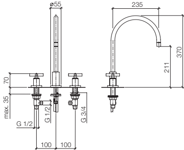
20 815 892 Three-hole mixer, 9 1/4" spout projection Batteria tre fori, sporgenza 9 1/4" Grifo mezclador con tres orificios, saliente 9 1/4"
