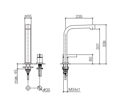
32 800 795 Two-hole mixer with individual flanges, 9 1/4" spout projection Miscelatore monocomando a due fori con rosette separate, sporgenza 9 1/4" Grifo mezclador con dos orificios con rosetas separadas, saliente 9 1/4"
