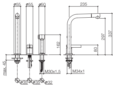
32 800 790 + 27 719 970 Two-hole mixer with individual flanges and handspray set, 9 1/4" spout projection Miscelatore monocomando a due fori con rosette separate e con gruppo doccetta lavello, sporgenza 9 1/4" Grifo mezclador con dos orificios con rosetas separadas y juego de grifo para cocina, saliente 9 1/4"
