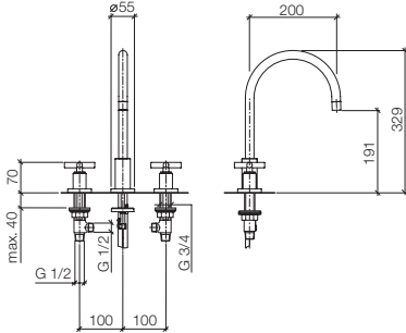
20 712 892 Three-hole mixer, 7 7/8" spout projection Batteria tre fori, sporgenza 7 7/8" Grifo mezclador con tres orificios, saliente 7 7/8"
