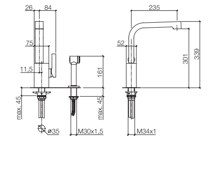
33 826 795 + 27 714 970 Single-lever mixer with handspray set, 9 1/4" spout projection Miscelatore monocomando con gruppo doccetta lavello, sporgenza 9 1/4" Mezclador monomando con juego de grifo para cocina, saliente 9 1/4"
