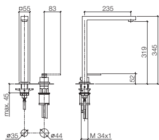
32 800 680 Two-hole mixer with individual flanges, 9 1/4" spout projection Miscelatore monocomando a due fori con rosette separate, sporgenza 9 1/4" Grifo mezclador con dos orificios con rosetas separadas, saliente 9 1/4"
