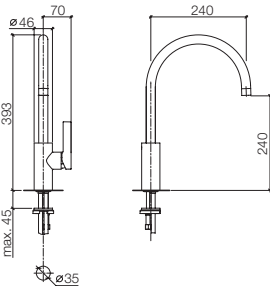
33 816 875 / 33 816 876 Single-lever mixer, 9 1/2" spout projection Miscelatore monocomando, sporgenza 9 1/2" Mezclador monomando, saliente 9 1/2"
