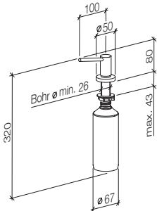
82 435 970 Deck-mounted liquid soap dispenser with flange Dispenser per detersivo liquido da incasso con rosetta Dosificador de lavavajillas encastrable con roseta
