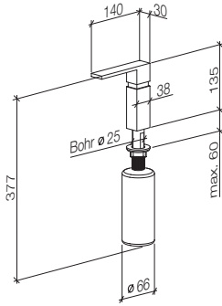
82 427 970 Deck-mounted liquid soap dispenser without flange Dispenser per detersivo liquido da incasso senza rosetta Dosificador de lavavajillas encastrable sin roseta
