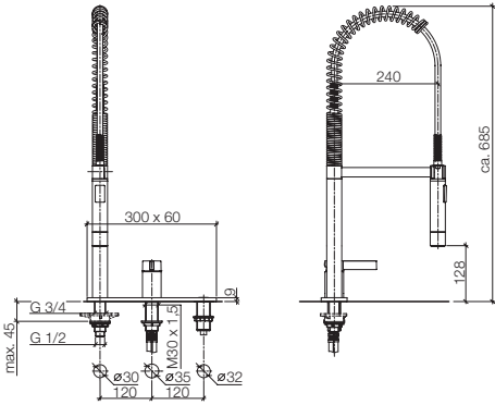
37 859 875 PREP SET Profi two-hole mixer, 9 1/2" spout projection, with Air Switch (operating button) // Miscelatore monocomando a due fori pro- fessionale, sporgenza 9 1/2", con Air Switch // Grifo mezclador profesional con dos orificios, saliente 9 1/2", con Air Switch
