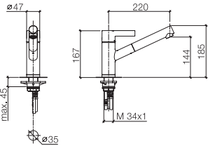
33 840 760 Single-lever lavatory mixer with pull-out spout, 8 5/8" spout projection Miscelatore monocomando con elemento bocca estraibile, sporgenza 8 5/8" Mezclador monomando con pieza final estraible, saliente 8 5/8"
