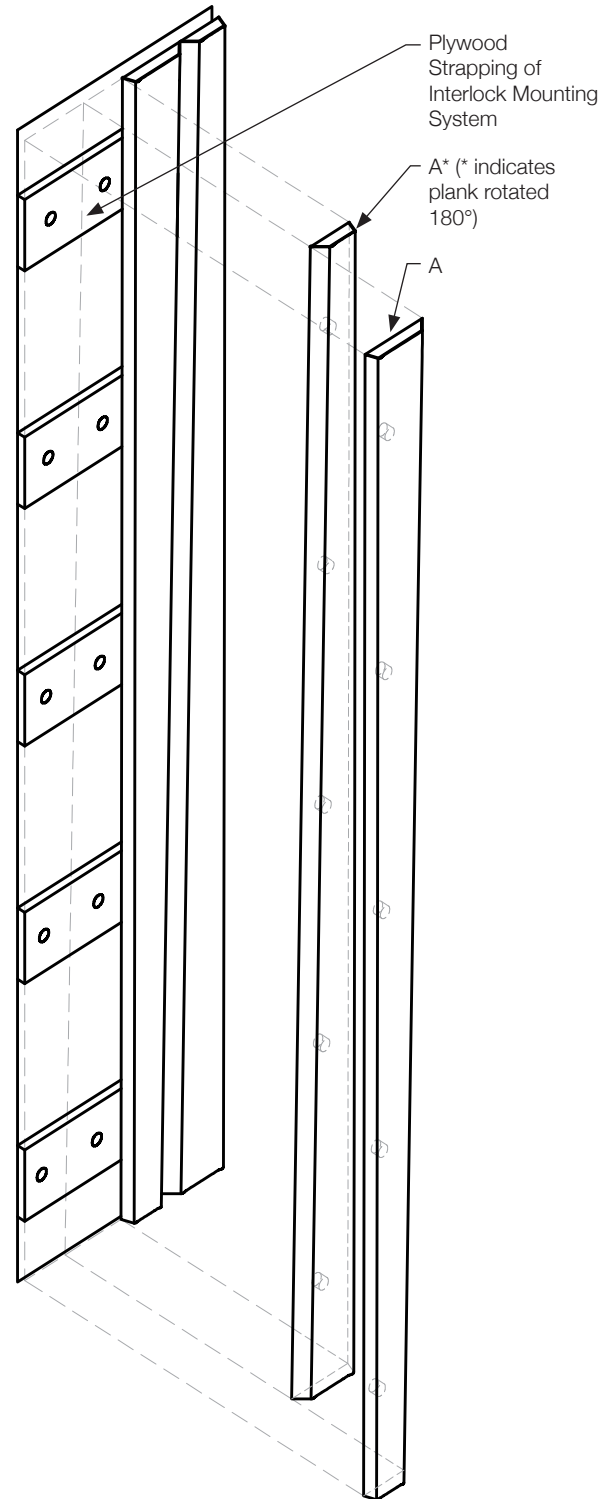
3 Exploded Axonometric Scale: 3/4" = 1'-0"
