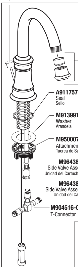
M964097-YYY0A Lift Rod and Knob Varilla de Drenaje y Perilla
