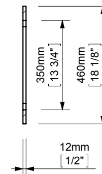
SECCIÓN A-A
