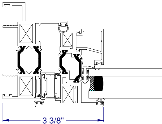
③ VENT JAMB
