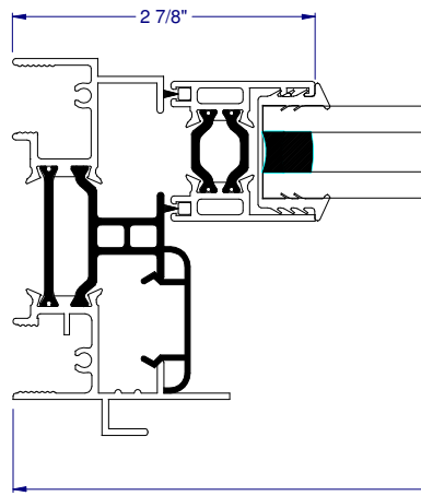
③ LEFT JAMB
