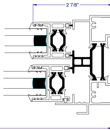
④ RIGHT JAMB
