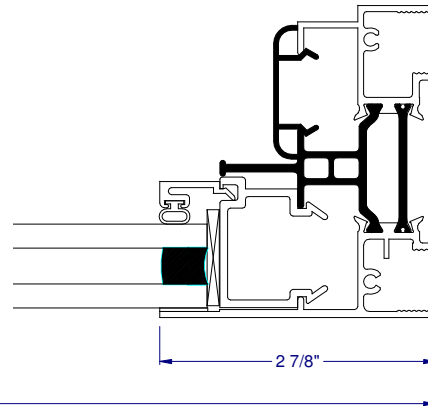
④ RIGHT JAMB
