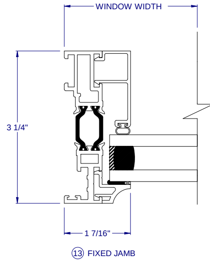
⑬ FIXED JAMB
