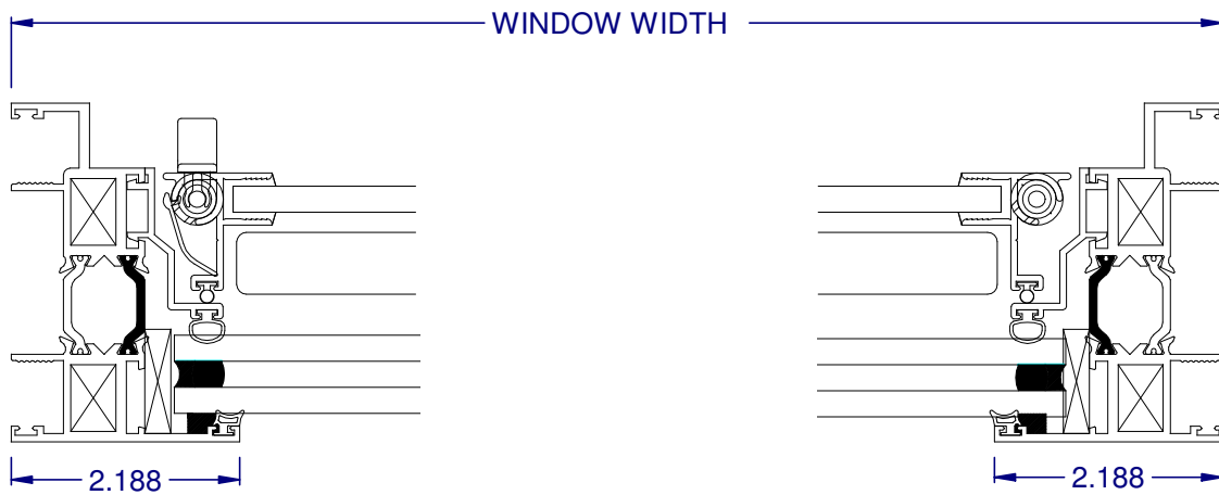
⑥ HORIZ. INTEGRAL MULLION
