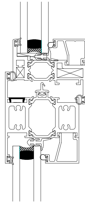
⑥ HORIZ. INTEGRAL MULLION
