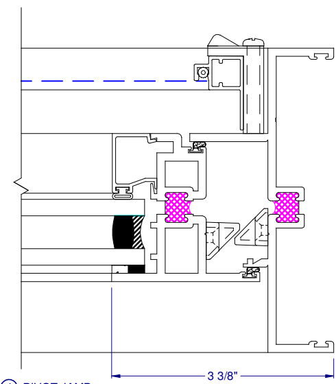
④ PIVOT JAMB
