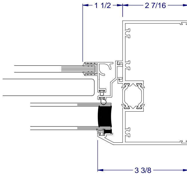
④ FIXED JAMB
