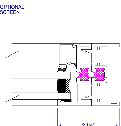
⑯ FIXED JAMB
