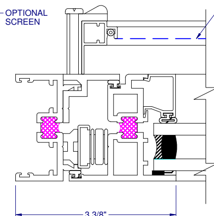
⑭a VENT JAMB
