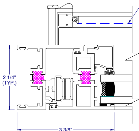
⑭ VENT JAMB
