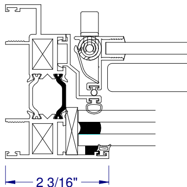
③ FIXED JAMB
