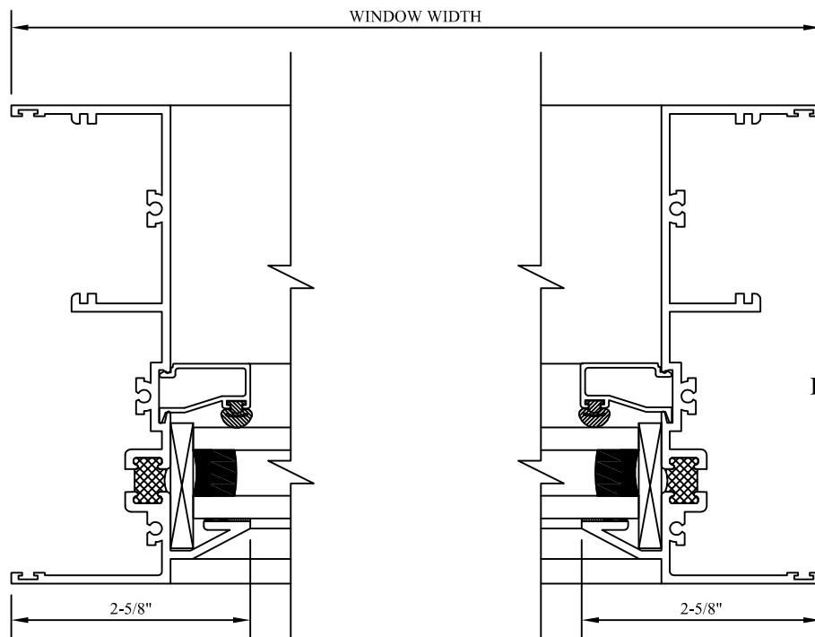
27 LEFT JAMB
