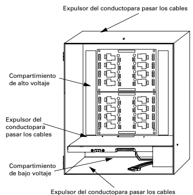
Recinto tamaño 16 con alto voltaje
