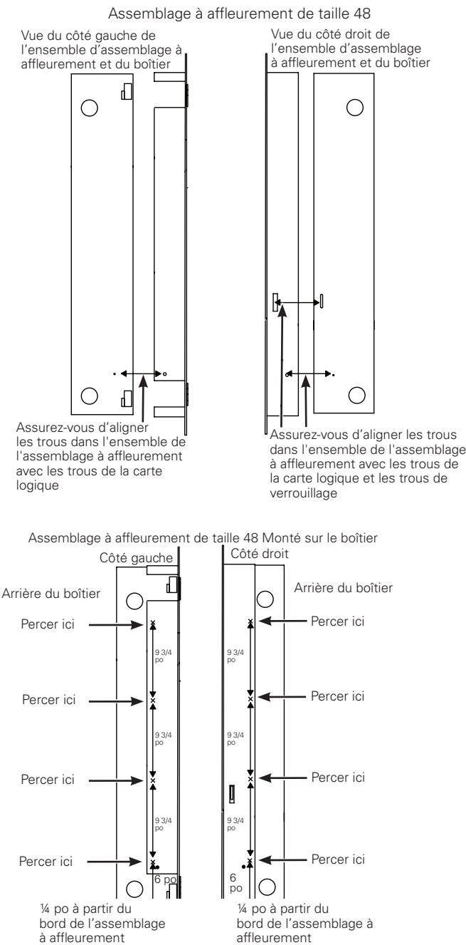
Figure 3. Boîtier de taille 48
