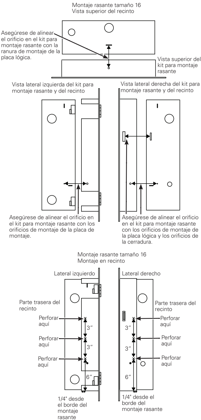
Figura 1. Recinto envolvente tamaño 16
