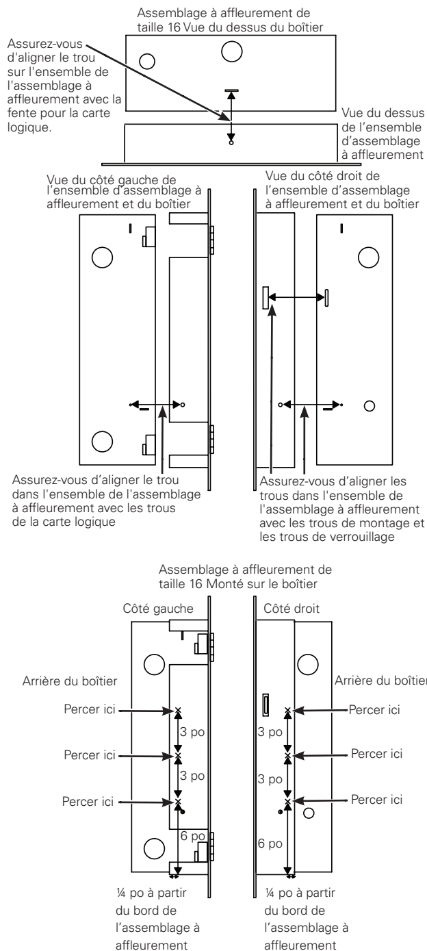
Figure 1. Boîtier de taille 16
