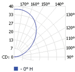
S.7006W - 3000K - 80 CRI
