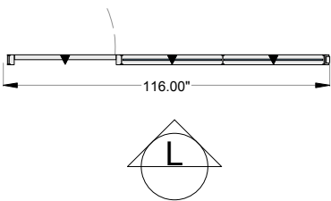
Elevation L
