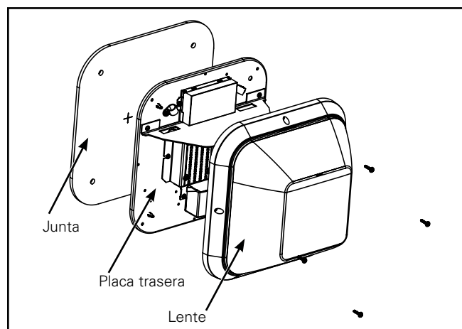
Figura 3. Instalación de la unidad plana
