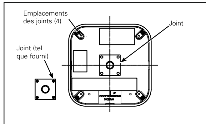
Figure 7 Emplacement du boîtier moulé peu profond
