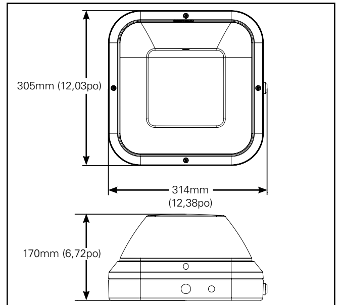
Figure 2 Modèle à boîtier peu profond
