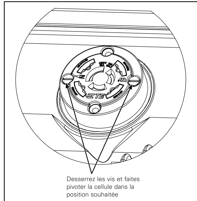
Figure 2. (À 7 BROCHES)
