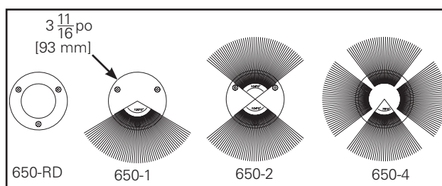
Figure 2. Option de garniture avec distribution de lumière différente
