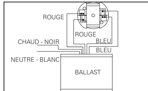
Figure 2. Schéma de câblage
