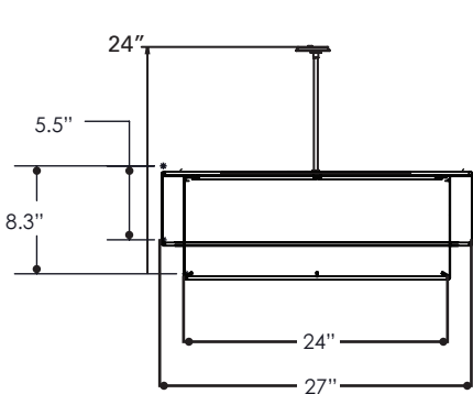
143-24-P1S (SINGLE STEM)
