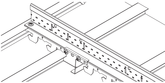
Retaining flange edge
