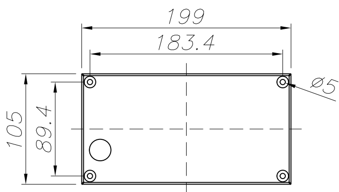
PLANTILLA DE INSTALACIÓN INSTALLATION TEMPLATE
