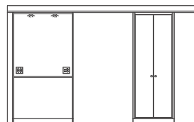
WALL UNIT HUTCH AND WARDROBE 12' TD22144WU3 D18 W144 H89.25 12' TD28144WU3 D24 W144 H89.25
