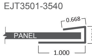
Edge J-Trim
