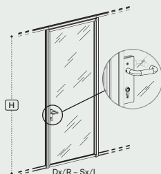
Porta anta battente vetro telaio slim /Glass hinged glass door, slim frame
