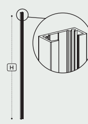
Profilo terminale /Terminal profile
