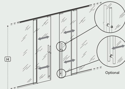
Porta scorrevole doppia anta in vetro /Double sliding glass door
