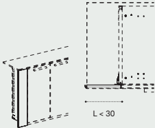
Fascia di tamponamento /Filler
