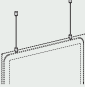
300.KT.05.00 Variante per fissaggio a soffitto con cavi /Ceiling fixing variant with cables
