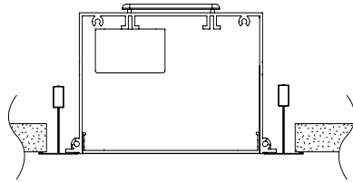
TB 15/16" + 9/16" T-BAR
