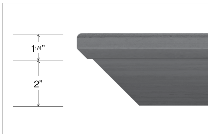
Edge Profile
