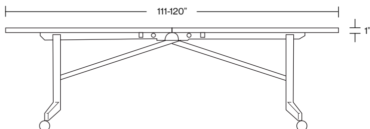
Tubular Base
