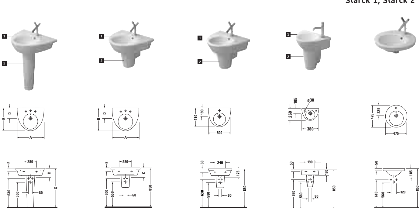
A B C D E F G 650 mm 650 510 205 220 75 630 550 600 mm 600 500 200 225 70 630 550 550 mm 550 470 200 225 60 630 550 A B C D E F G 650 mm 650 510 205 220 75 630 550 600 mm 600 500 200 225 70 630 550 550 mm 550 470 200 225 60 630 550
